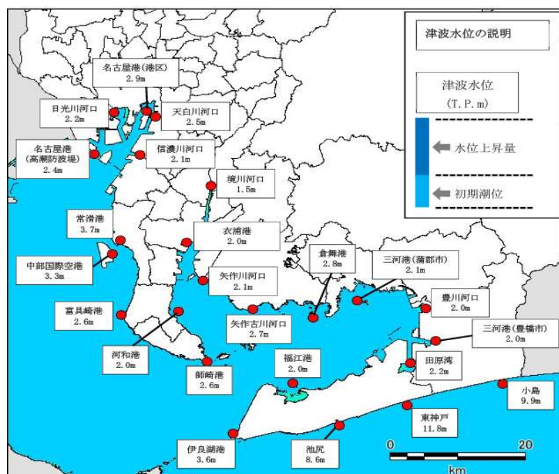
図-15 代表地点における津波水位予測図
